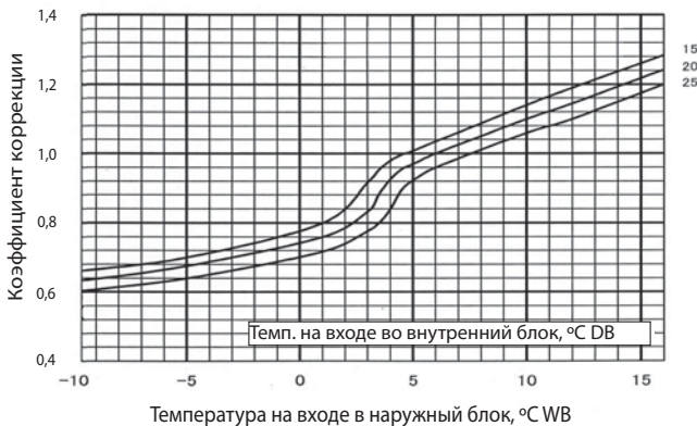
Рис. 4-3. Теплопроизводительность
