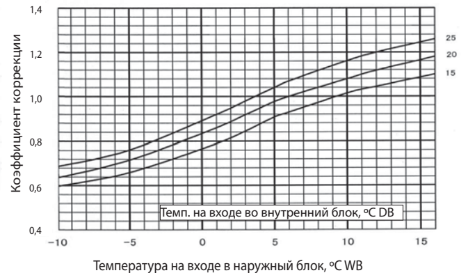
Рис. 4-4. Потребляемая мощность в режиме обогрева
