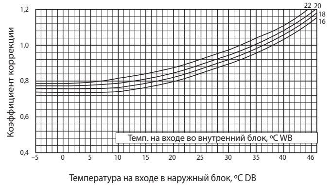
Рис. 4-2. Потребляемая мощность в режиме охлаждения
